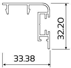
DIE No. W72204 Clip-On Interlocker
