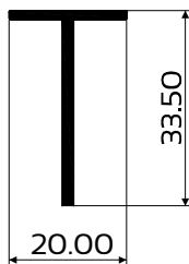
DIE No. W32846 Astragal T
