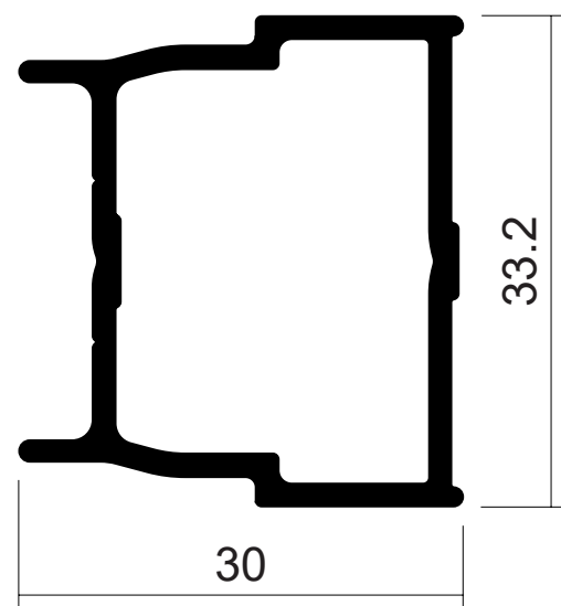
DIE No. W59151 | Guardian Jamb
