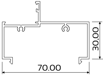
DIE No. W70968 Swift 30.5 Frame 70mm
