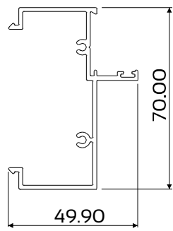
DIE No. W70963 Case 28 Frame 70mm
