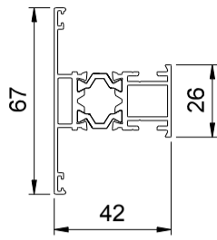
EDGE MULLION C0003
