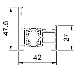
EDGE FRAME EQUAL LEG C0001
