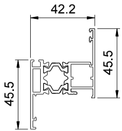
EDGE SASH C0002
