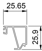
EDGE BEAD MULTI 13mm GAP C0004
