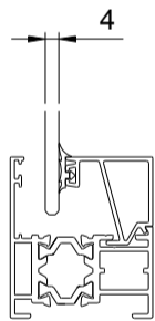
EDGE BEAD MULTI 13mm GAP C0004
