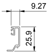
EDGE BEAD DOUBLE GLAZING C0005
