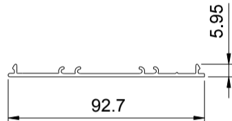
MULTI FIXING LUG W30607
