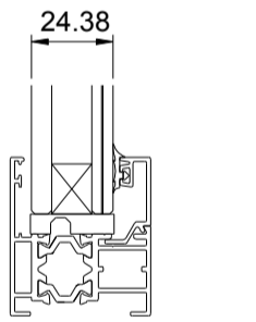
EDGE BEAD DOUBLE GLAZING C0005
