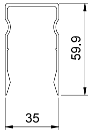
STIFFENER CAP W29824
